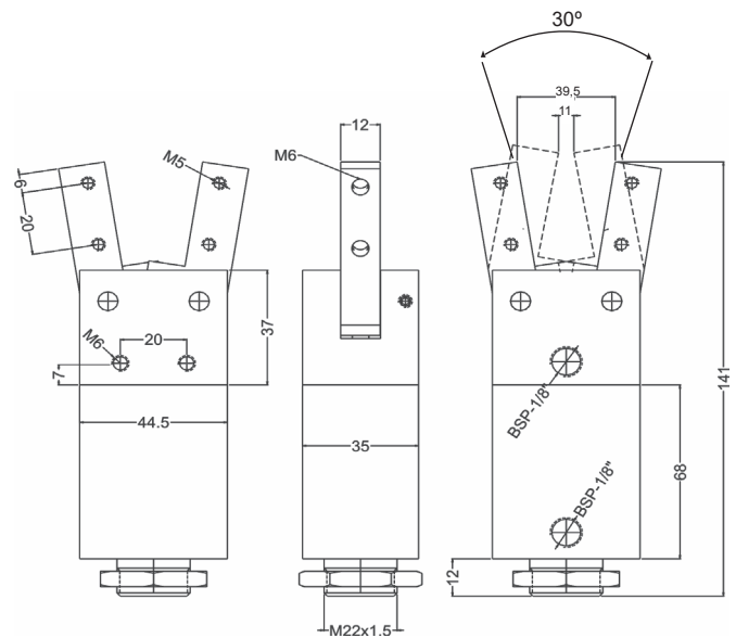
Garra Ø32
