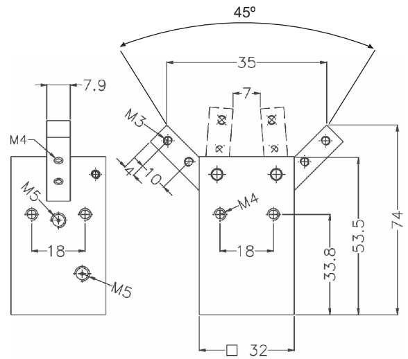
Garra Ø20
