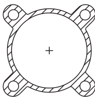
Tubo Mickey Mouse Para os cilindros de diâmetros de 32,40,50,63,100 e 125 Modelo "P"
