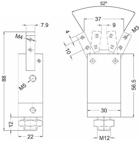
Garra Ø16
