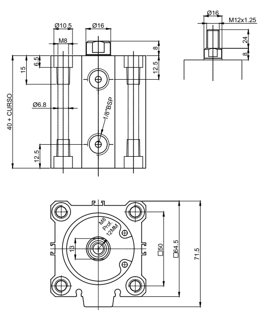
Cilindro Ø 50
