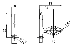
SUPORTE CENTRAL - REF.: 1100-40U (MATERIAL: Alumínio)
