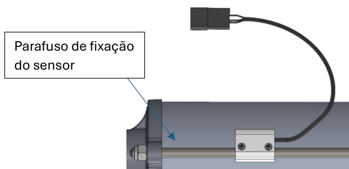
Figura 4 - Sensor magnético
