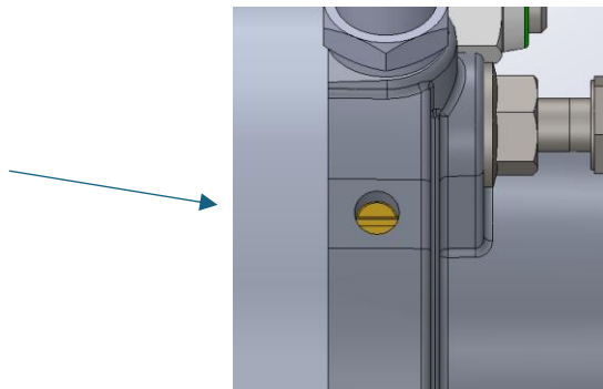
Figura 5 - Regulagem do amortecimento
