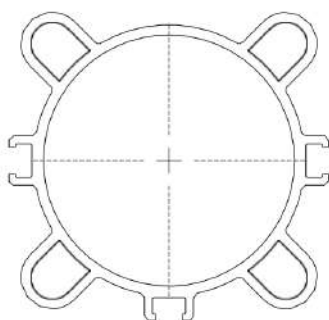
Tubo Perfilado para Tirante. Para os cilindros de diâmetros de 32, 40, 50, 63 e 100 Modelo "TA"
